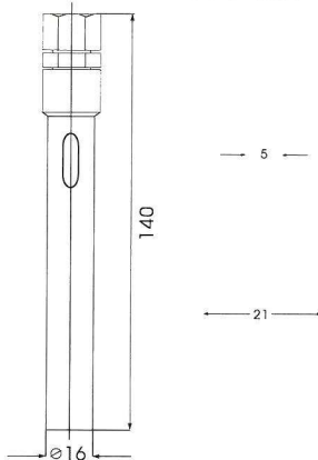
2-Stab Sondenkopf SK2/3-Stab Sondenkopf SK3 Sondenlänge 2 bzw. 3 mal 500 mm
