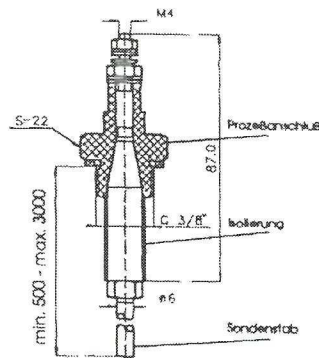
2-Stab Sondenkopf SK2/3-Stab Sondenkopf SK3 Sondenlänge 2 bzw. 3 mal 500 mm
