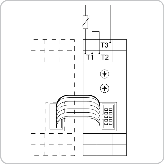
2-Leiter Messmethode
