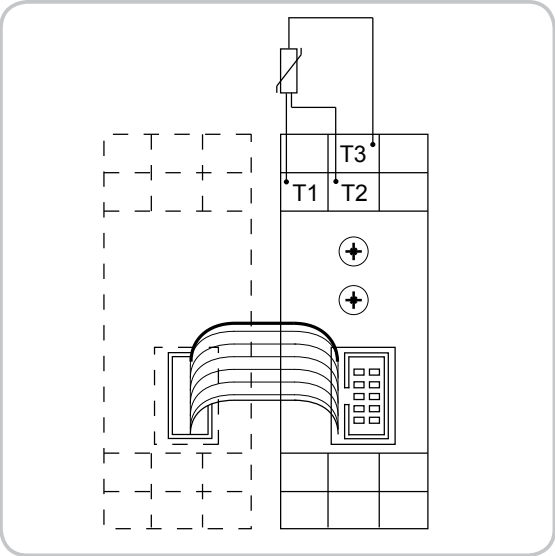
3-Leiter Messmethode
