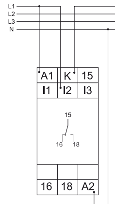
Range 1A con modulo alimentazione 230V AC
