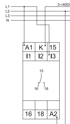
Range 5A con modulo alimentazione 400V AC
