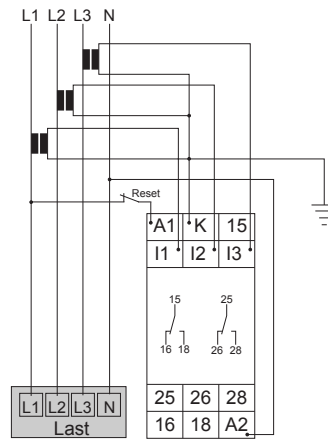
G2JM5AL20, Versorgung 230V AC mit Stromwandler und Fehlerspeicher
