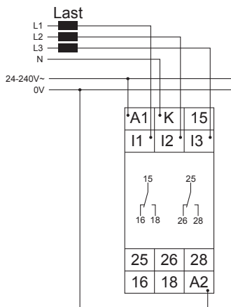
G2JM5AL20, Versorgung 24-240V AC/DC ohne Fehlerspeicher
