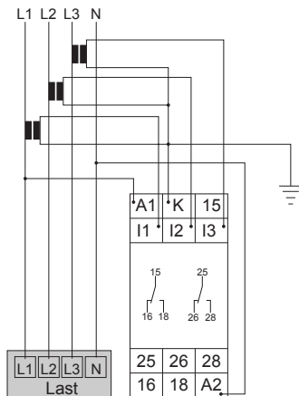
G2JM5AL20, Versorgung 230V AC und Stromwandler
